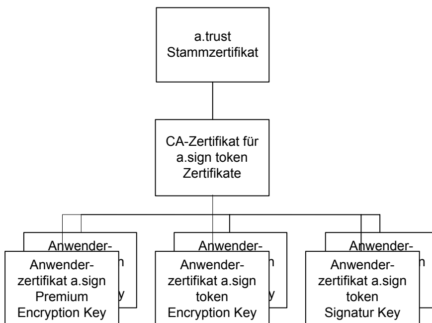
Abbildung 1 Zertifizierungshierarchie
